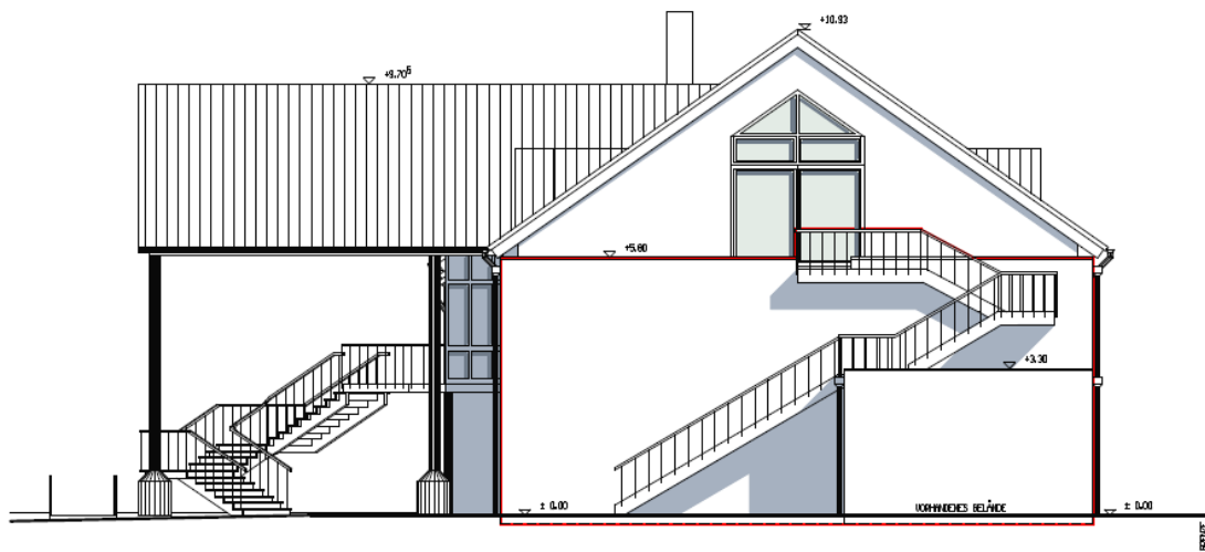
ANSICHT VON NORDWESTEN M 1:100
