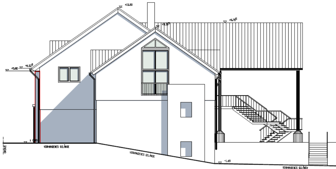
ANSICHT VON NORDWESTEN M 1:100
